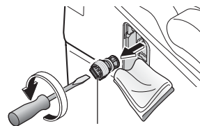
Ablaufventil mit Filter
